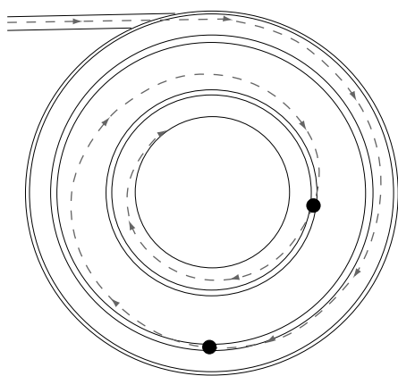
Figuur 1 Bovenaanzicht met de baan van de kogel door een Golden-Ten ketel. De kogel is afgebeeld op de plekken waar deze achtereenvolgens de 'observatiering' en de 'limietring' snijdt. Dit schema is ontleend aan de nota 'Golden Ten in perspectief' (1989) van de NSGT.
