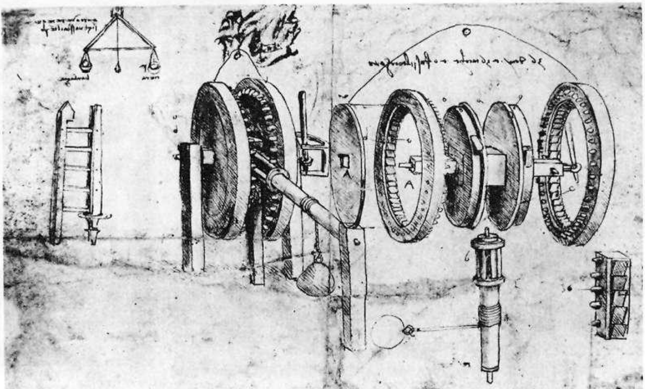
21. 'Vnterse of Prection*. Kadermechaniek van Leonardo da Vinci, ca. 1500. Links samengesteld, rechts in de onderdelen uit-clkaar-getekend.
